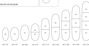
Electrical Module
